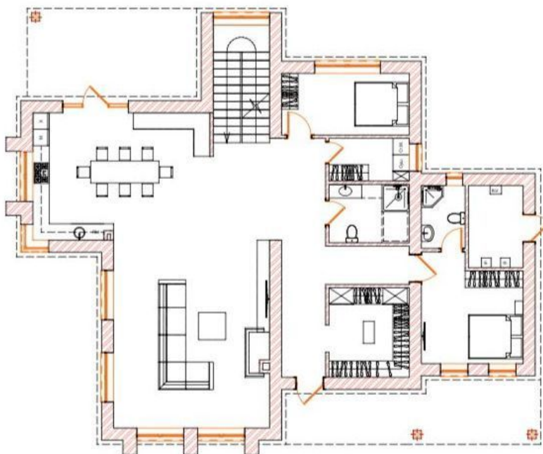
План с мебелью на отм. +0.000
